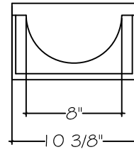
Vue du dessus/ Top View
