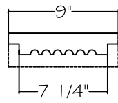
Vue du dessus/ Top View
